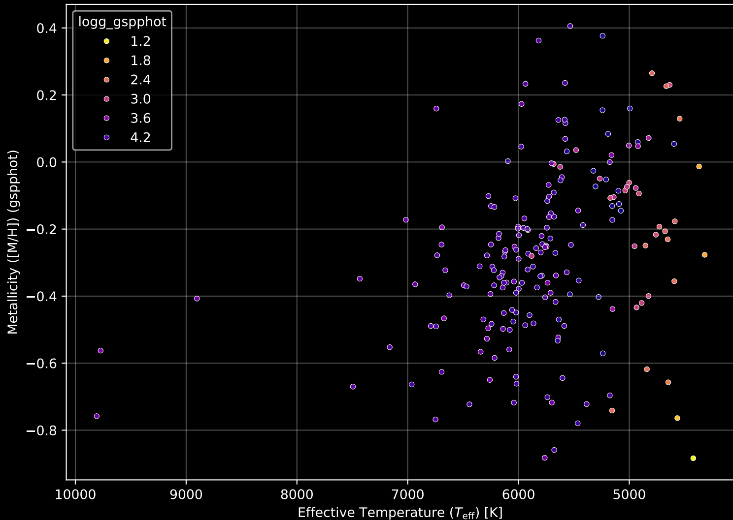
GALAH DR4 Field: [7139] Stellar Population Parameters (n= 196)
