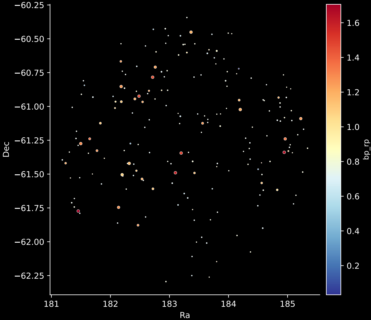
GALAH DR4 Field: [7139] Stars: 196
